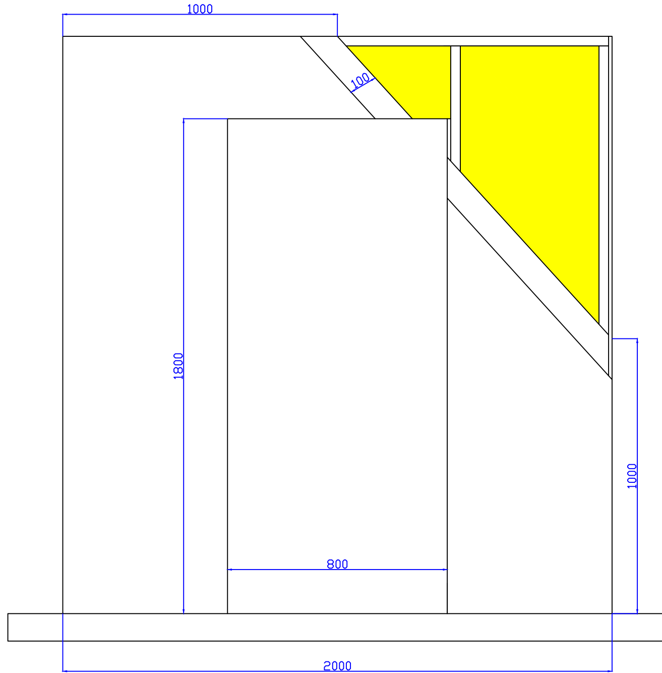
ELEVATION B
